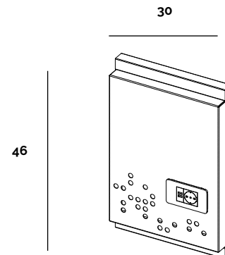
SCHIENALE ELETTRICO / ELECTRIC BACKREST
