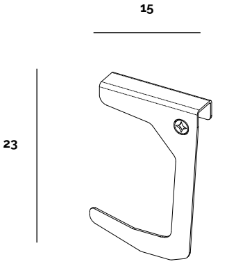
GANCIO BICI / HOOK FOR BIKE
