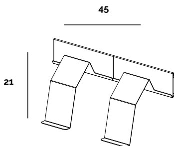
KIT PORTACASCHETTO / HELMET HOLDER
