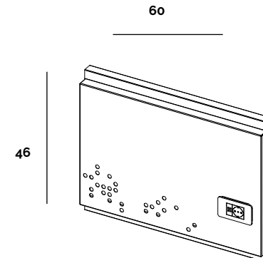
SCHIENALE ELETTRICO / ELECTRIC BACKREST
