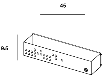
GANCIO BICI / HOOK FOR BIKE
